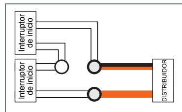
CABLEADO EN SERIE para pares simultáneos o pares de doble salida
