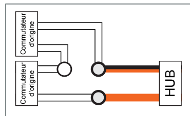
CÂBLAGE EN SÉRIE Paire de portes à ouverture simultanée ou à deux battants
