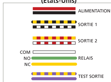
Faisceau de câblage antérieur (États-Unis)
