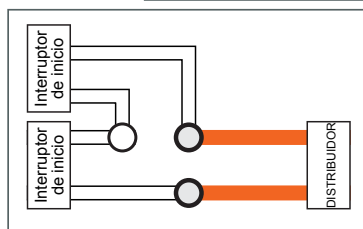
CABLEADO EN SERIE para pares simultáneos o pares de doble salida
