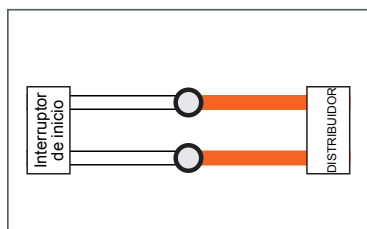
CABLEADO NORMAL para puertas individuales
