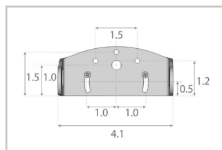
Dimensions du support
