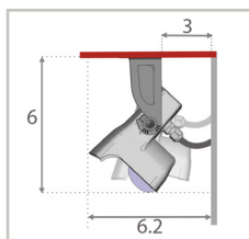
Installation au plafond
